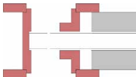
Waagrechter Schnitt In der Wand laufend - Taschenverkleidung bauseits Empfehlung Taschenbreite: Türstärke +10 mm
