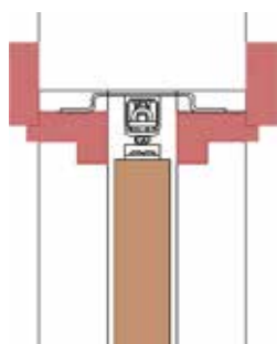
Senkrechter Schnitt In der Wand laufend mit abnehmbaren Blenden, Schiene vormontiert
