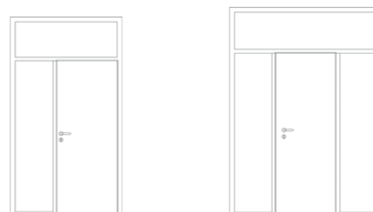
Feststehende Seitenteile mit Oberlicht
